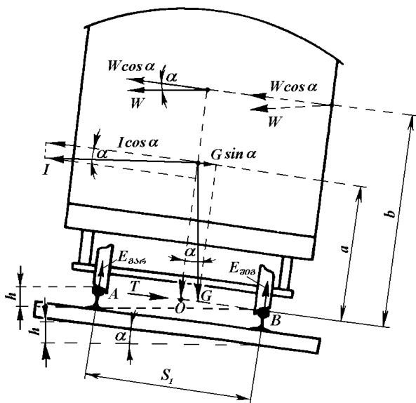
ნახ. 2. მრუდებში გარე რელსის შემადგენლისა და შიგა რელსის ეკვივალენტური მოდელის სქემა.
