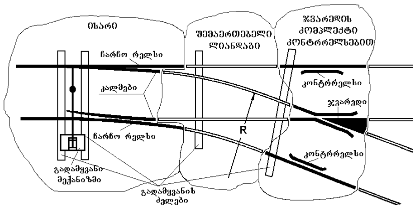
ნახ.6. ერთმაგი ისრული გადაყვანის სქემა
