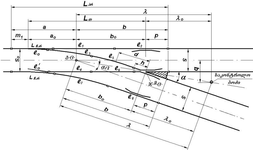
ნახ.13. ისრული გადამევანის ძირითადი გეომეტრიული ზომები
