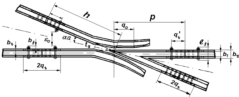
ნახ.12. ჯვარელის სიგრძის განსაზღვრის სქემა
