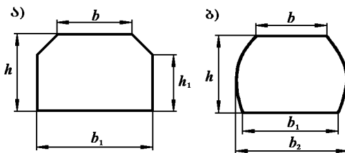
ნახ.15. გადამყვანის ხის ძელების განივი კვეთის ფორმები: ა) ჩამოგანილი; ბ) ჩამოუგანავი
