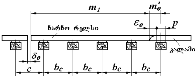
ნახ.9. m_1 მანძილის განსაზღვრის სქემა
